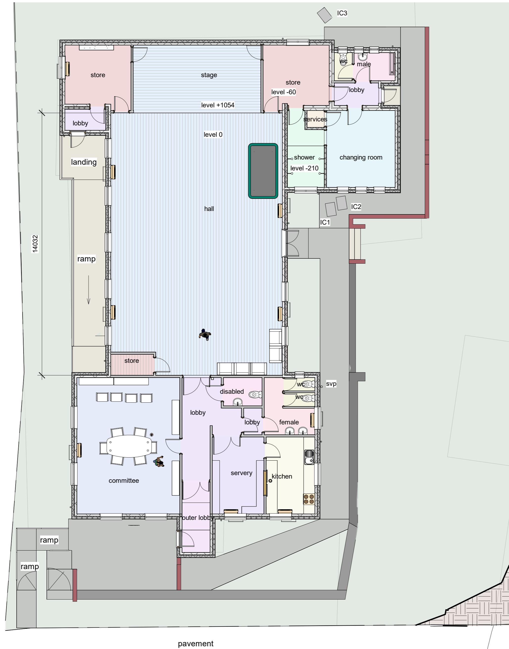
1 0_grd FFL Existing 1 : 100
